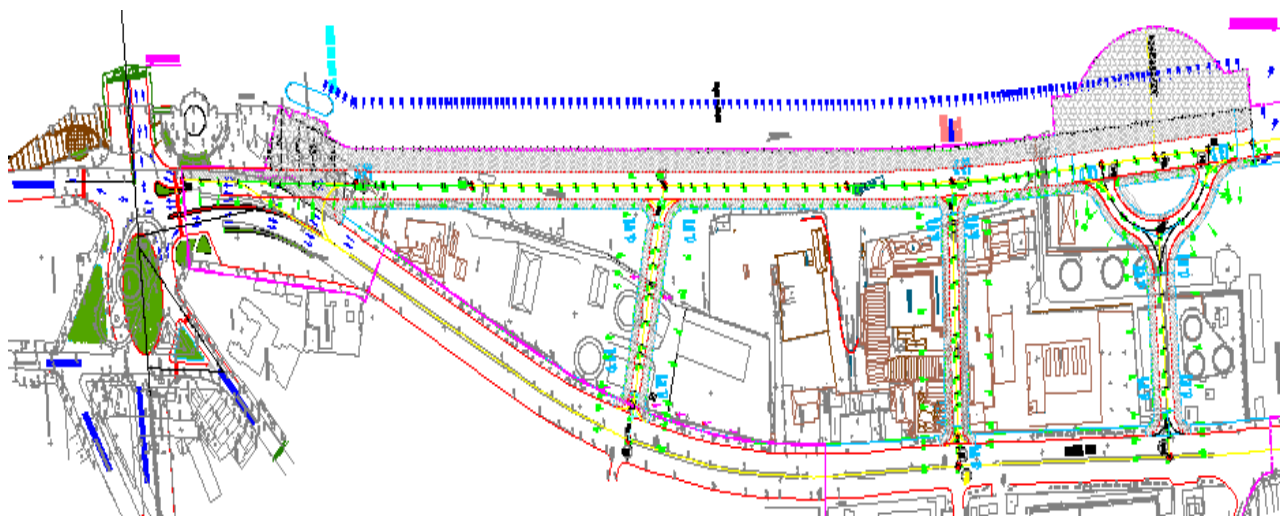
Bình đồ tổng thể khu phức hợp TM-DV phường Bình Hiên- Bình Thuận - Tp Đà Nẵng
